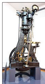
Fig. 64 - Primeiro Motor Diesel de 1893 (Fonte: [73]).
