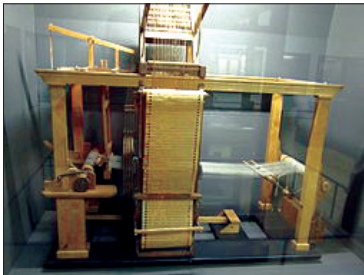
Fig. 3 - Tear de Basile Bouchon 1725 (Fonte: [5]).
