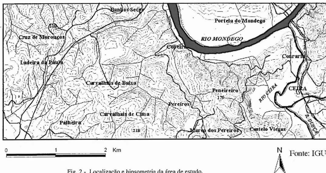
Fig. 2 - Localização e hipsometria da área de estudo.
