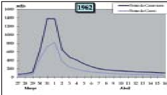
Fig. 5 - Evolução do caudal médio diário durante a cheia de Abril de 1962 (Fonte: PEROSA e COSTA, 1999).
