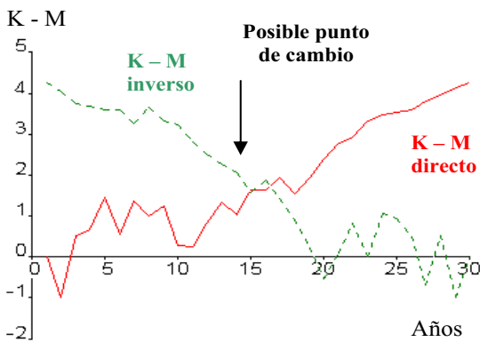
Fig. 9 A - Comportamiento del estadígrafo de Mann - Kendall (directo e inverso) . Duración de la temporada de días con CCI_{sv} - todas las categorías. Santiago de las Vegas. 1975- 2004.
