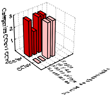
Fig. 11 - Distribución de CCIsv y CCIcv en la ciudad. 4 de agosto de 1987.
