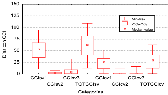
Fig. 3 - Estadígrafos representativos de CCI. Stgo. de las Vegas. 1975-2004.
