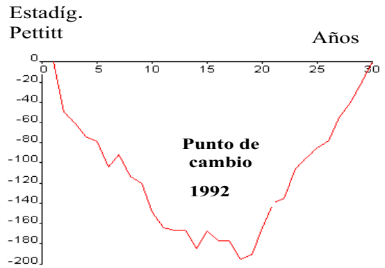
Fig. 9 B - Comportamiento del estadígrafo de Pettitt para la misma serie. Santiago de las Vegas. 1975-2004.
