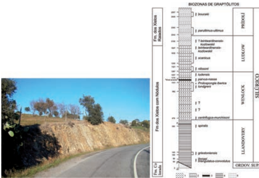
Fig. 2 – Secção do Silúrico da trincheira do km 102.15 da EN 258 (à esquerda) e respetivo log estratigráfico esquemático, com indicação das biozonas de graptólitos determinadas (à direita). Legenda do log – 1 – xistos cinzentos com finas intercalações quartzíticas, 2 – xistos negros, 3 – “nível amarelo” (? vulcânico), 4 – liditos e xistos negros, 5 – quartzitos.
