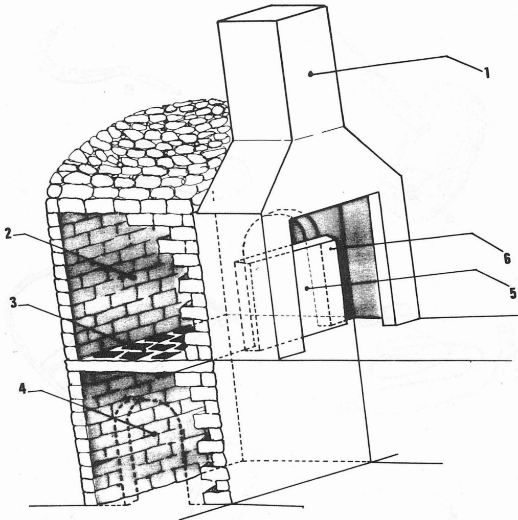
Fig. 5 — O forno. 1 — chaminé; 2 — sobrecéu; 3 — crivo com os olhais; 4 — caldeira ou fornalha; 5 — boca; 6 — tapadoiro.
