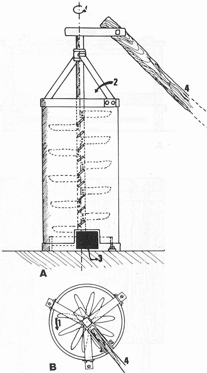
Fig. 4 — A maroma.
