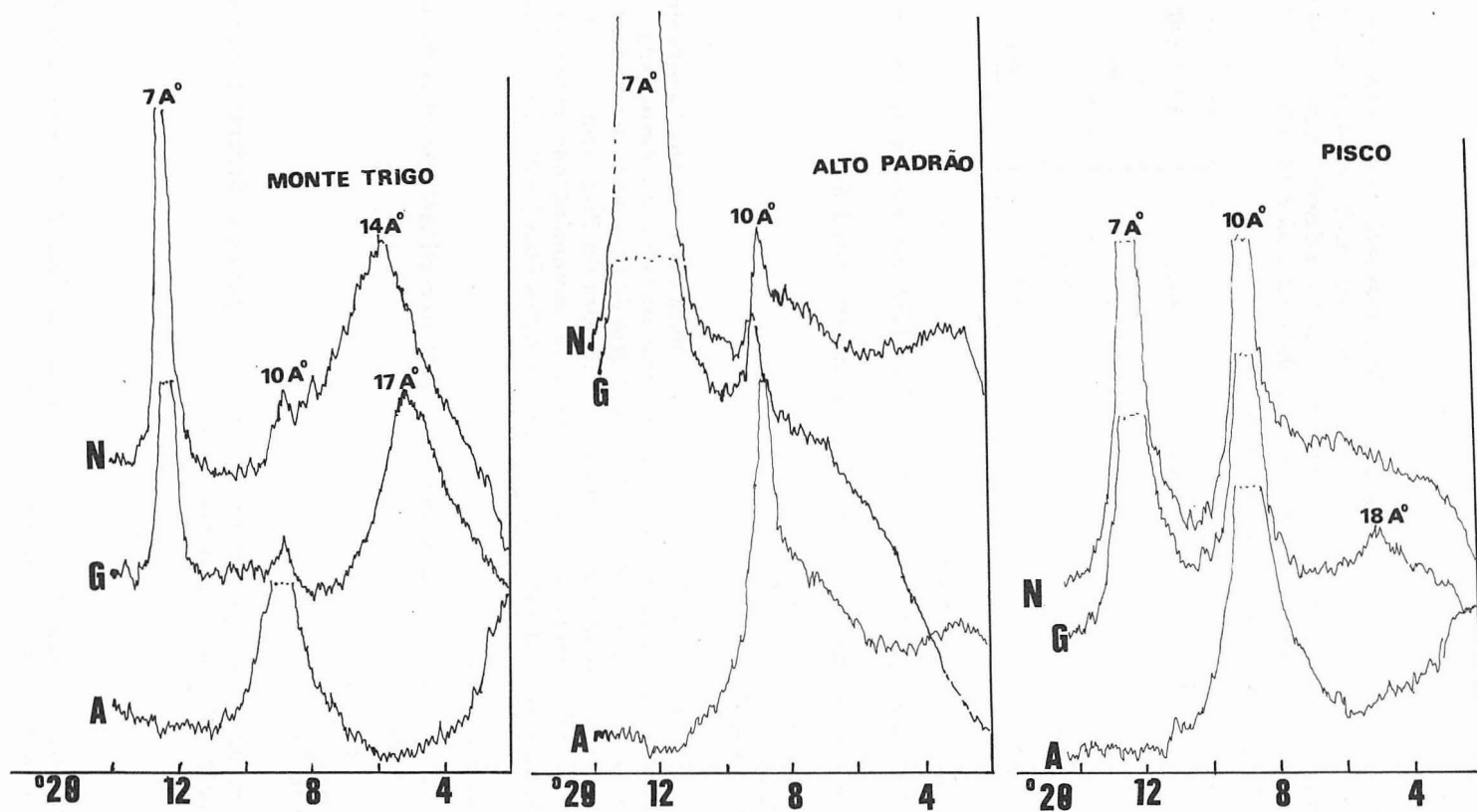
Fig. 1 — Difractogramas de fração argilosa ( <2 micra) obtidas em lâmina sedimentada. N — normal, G — glicolada e A — aquecida a 550^{\circ}\text{C} .
