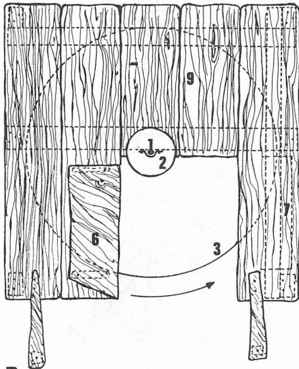
Fig. 3 — O torno.
